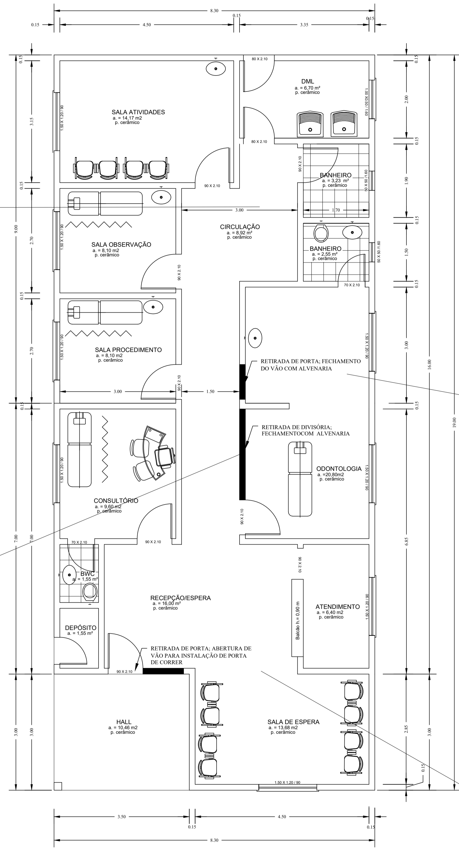
PLANTA BAIXA EXISTENTE ESCALA 1 : 50
