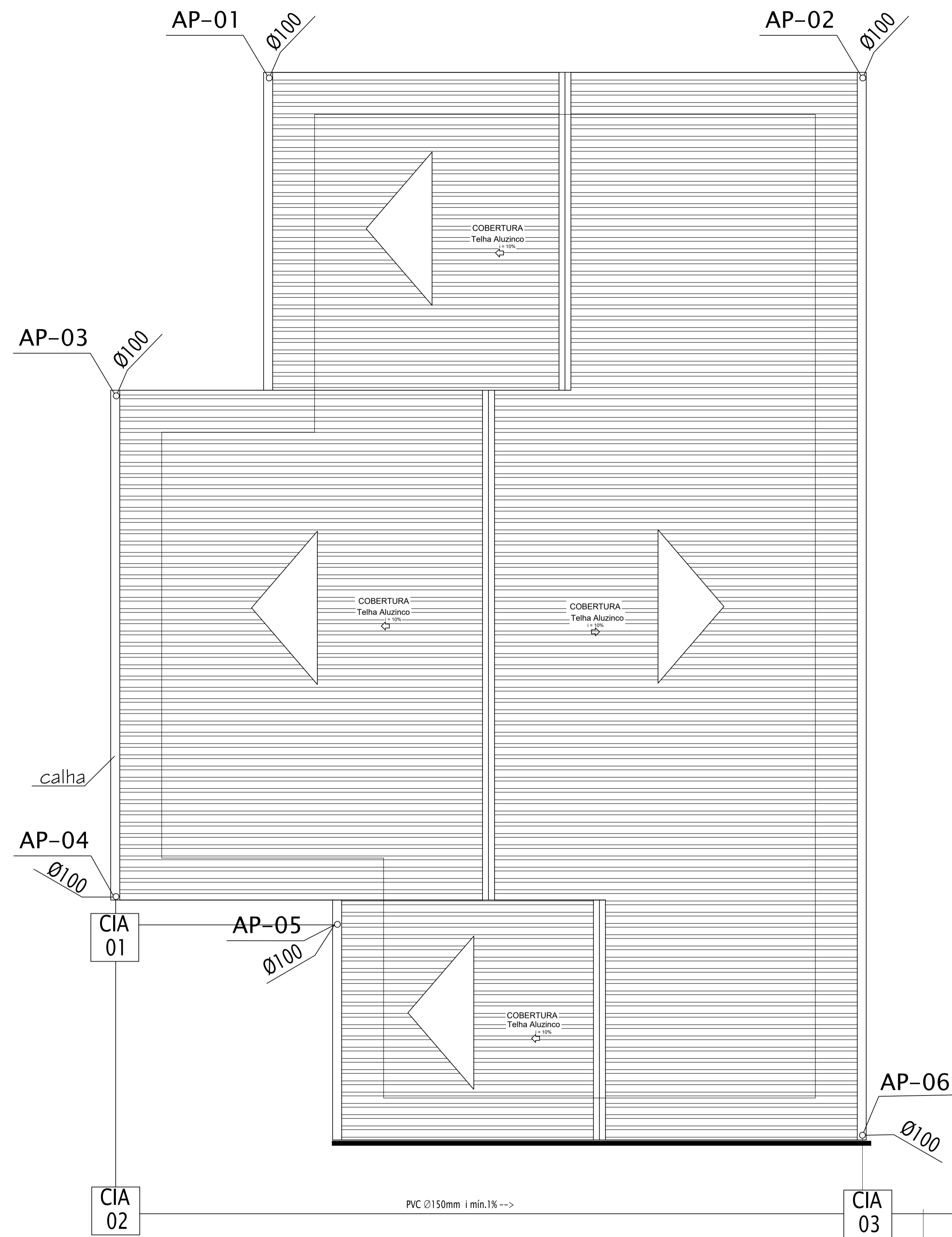
PLANTA COBERTURA - AGUAS PLUVIAIS ESCALA 1 : 50
