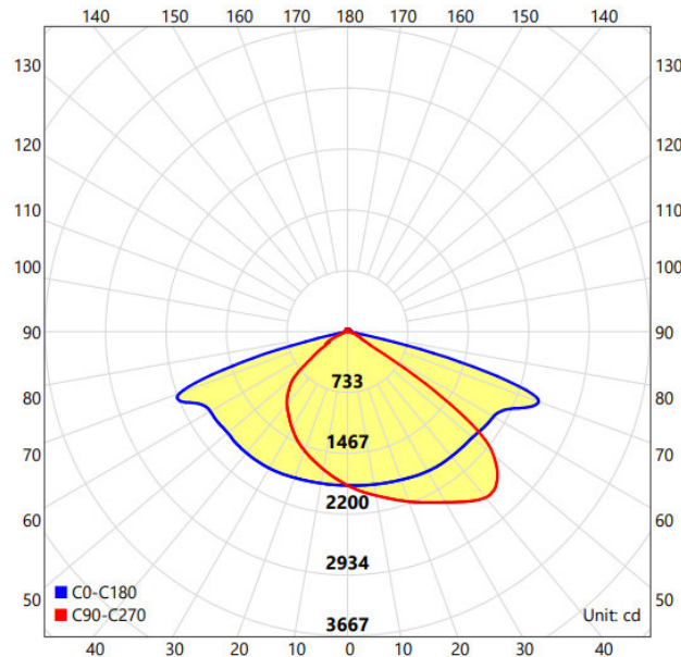
Figura 05 – Distribuição de intensidade luminosa
