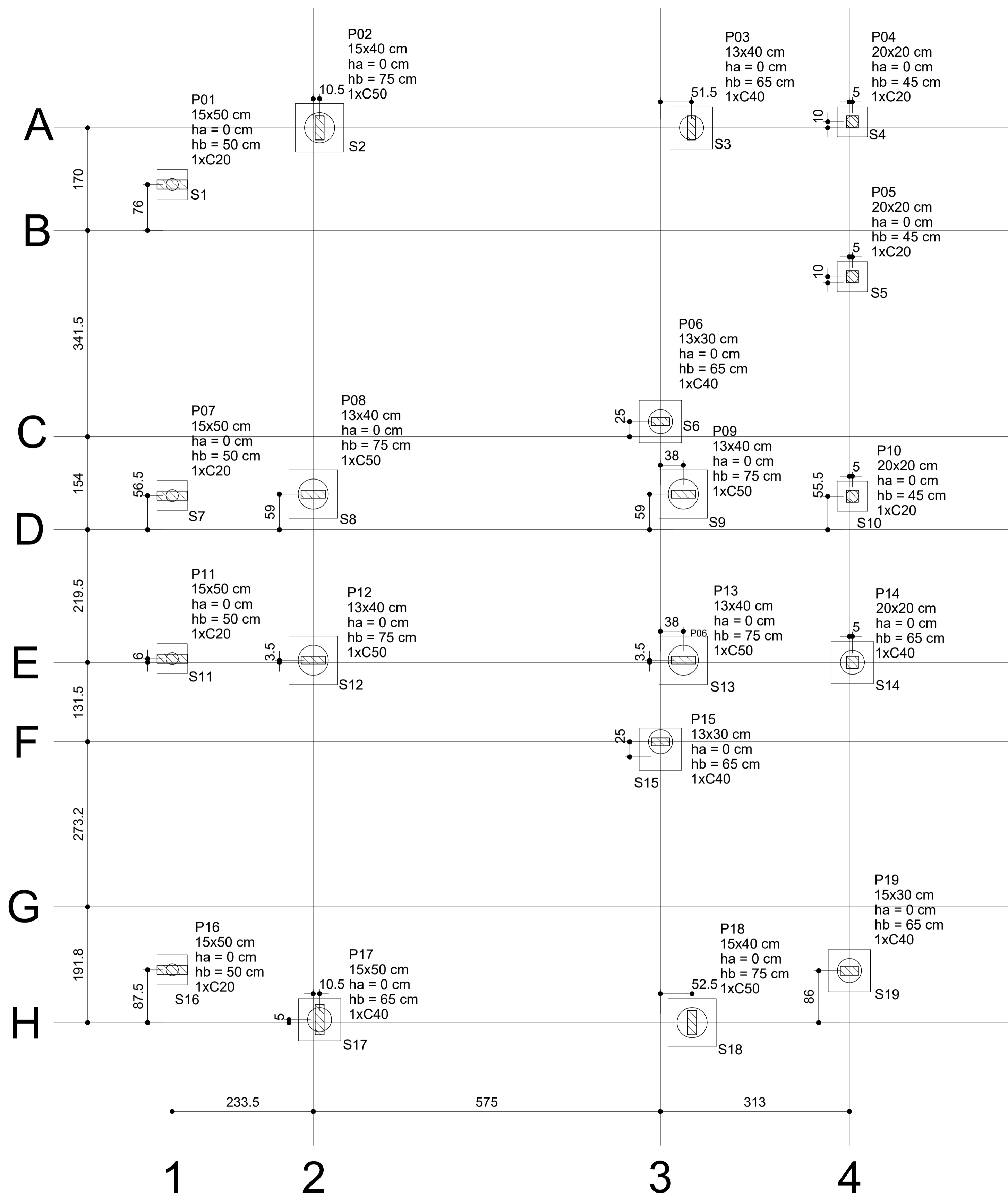
Planta de locação escala 1:75
