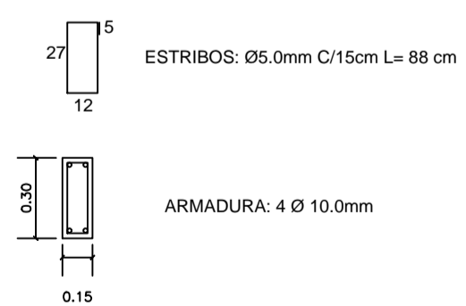
DET. VIGAS COBERTURA ESCALA 1:50
