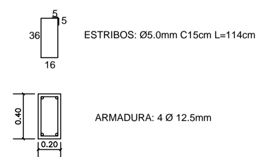
DET. VIGAS BALDRAME ESCALA 1:50
