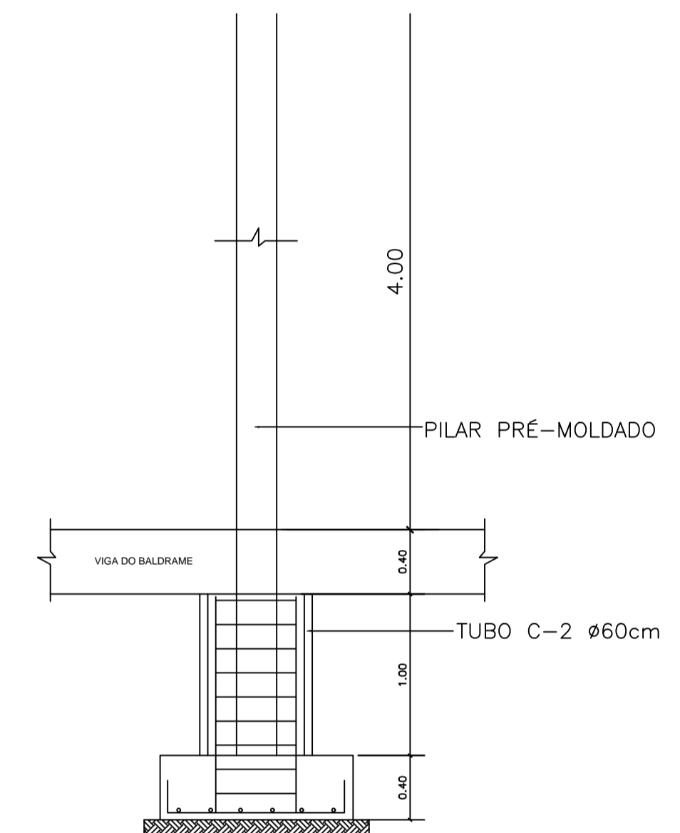
OBSERVAÇÕES: DIMENSÕES DOS PILARES: 23 x 40 cm DEVERÁ TER GARANTIA DO FABRICANTE CORTE AA - PILAR PRÉ-MOLDADO ( 25x ) ESCALA 1:25
