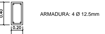
DET. VIGAS BALDRAME ESCALA 1:50
