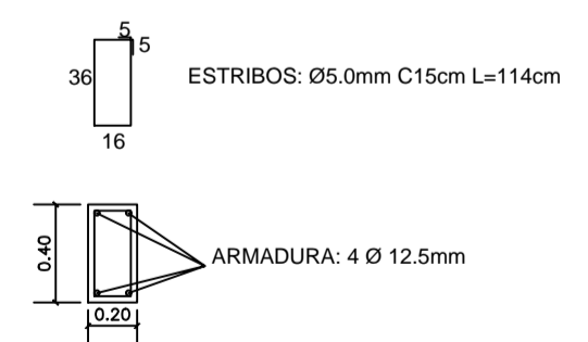
DET. PILARA MOLDADO "IN LOCO" (5X) ESCALA 1:50
