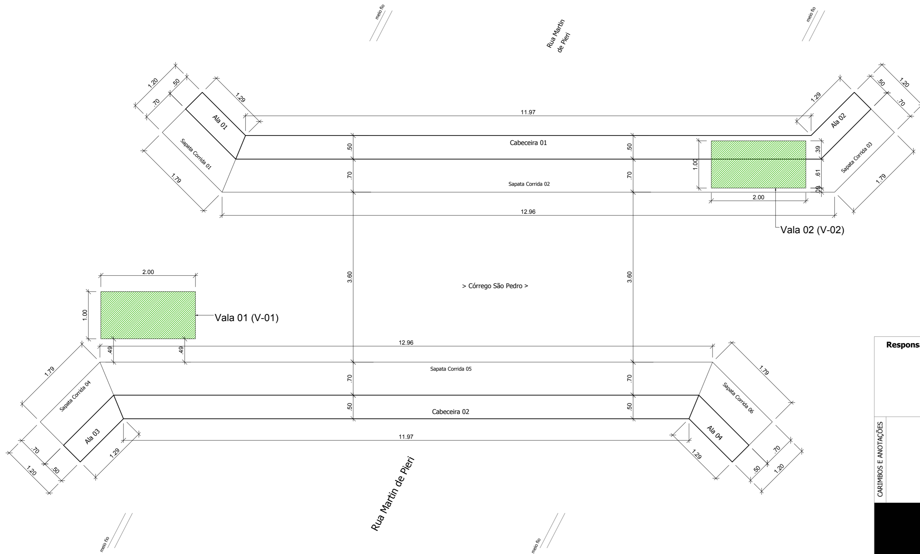
Croqui de Localização das Valas de Sondagem esc. 1/50
