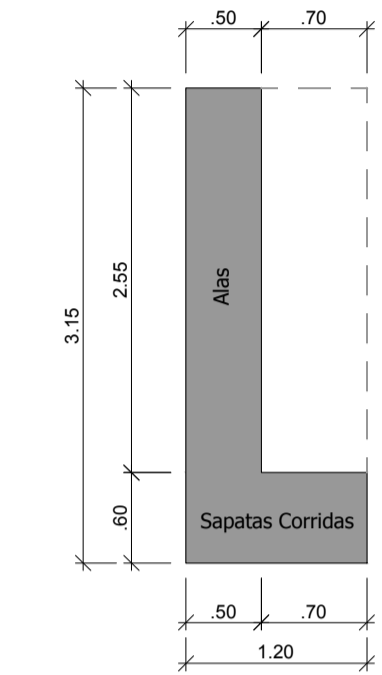
Corte Esquemático Alas esc. 1/50
