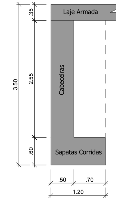
Corte Esquemático Cabeceiras esc. 1/50
