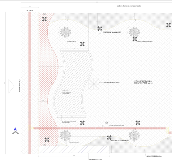
Planta baixa PRÉFABRICO 01 Área: 458,00 m² ESCALA 1/50
