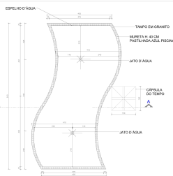
Planta baixa espelho d'água + capsa do tempo Área: 28,00 m² ESCALA 1/50
