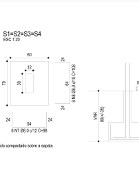
DETALHE VIGAS - BALDRAMES E FECHAMENTO ESCALA INDICADA V101 = V102 V103 = V104
