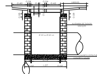
CORTE BB ESCALA 1/10
