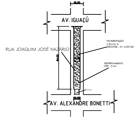
TRECHO 03: RUA JOAQUIM JOSÉ NAZÁRIO ENTRE AV. IGUAÇU E AV. ALEXANDRE BONETTI ESCALA 1/1.000
