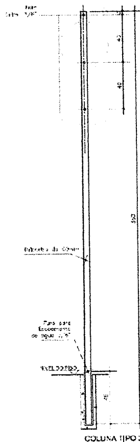
COLUNA TIPO 2
