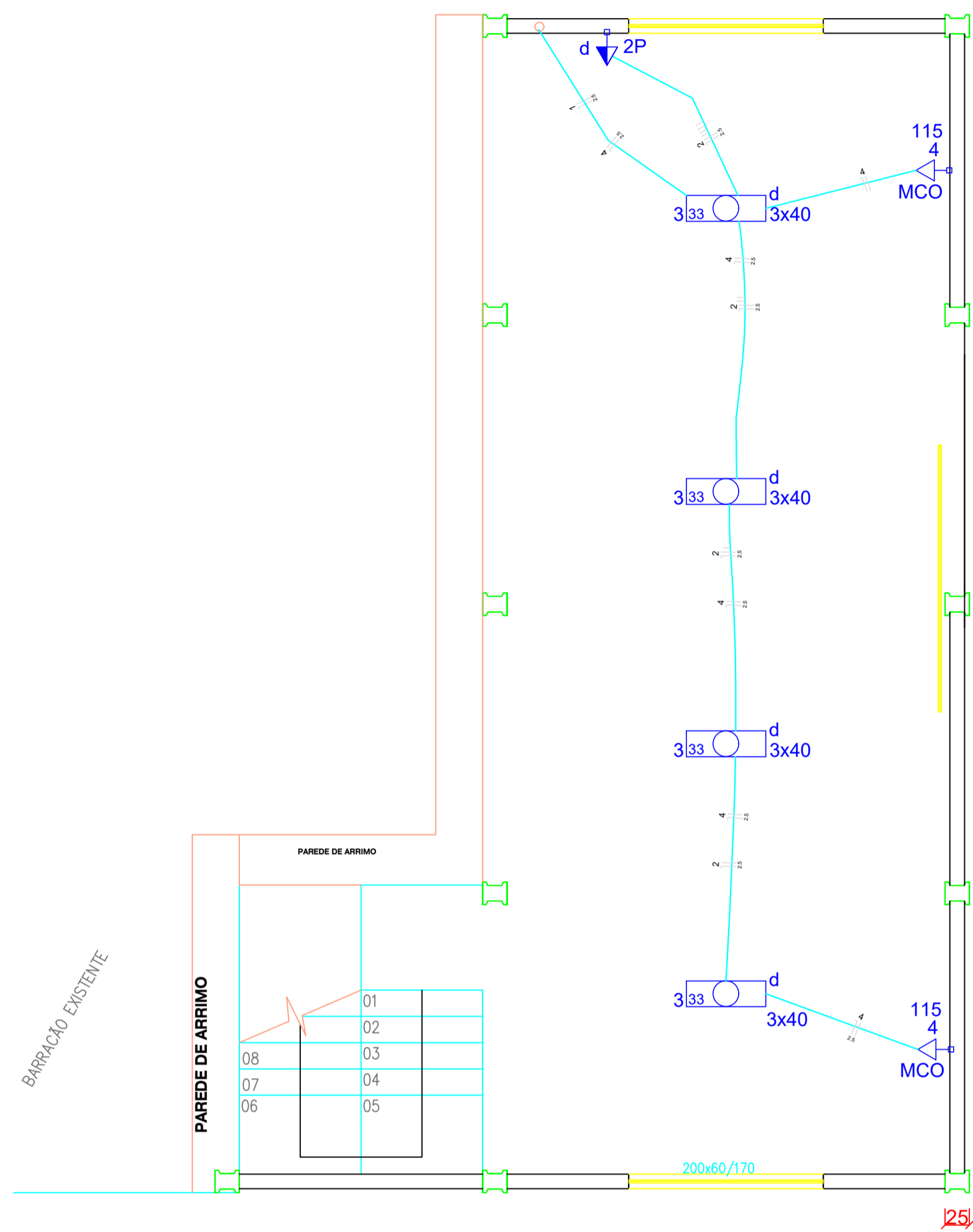
PLANTA BAIXA - SUB-SOLO ESCALA 1:50
