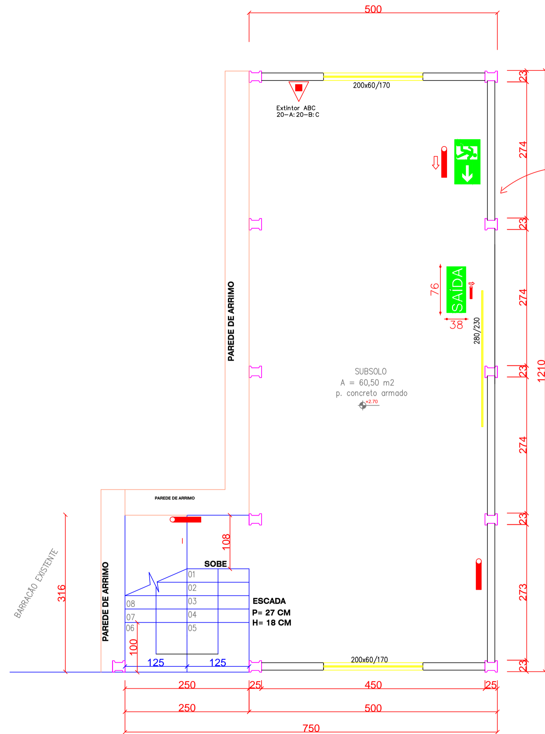
PLANTA BAIXA - SUB-SOLO
