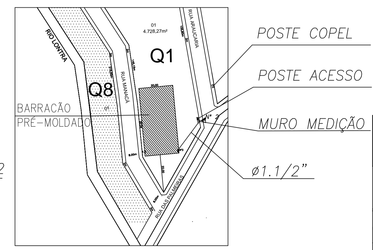
PLANTA DE SITUAÇÃO Escala 1/1000
